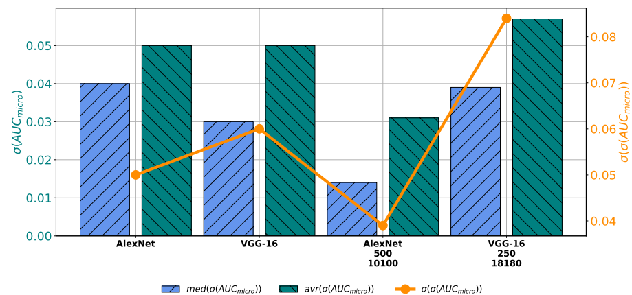
(b) \sigma(AUC_{micro})
