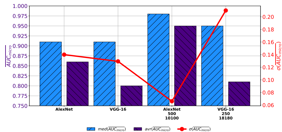
(a) AUC_{micro}
