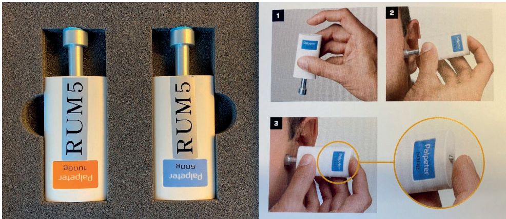
Slika 1. Palpater – algometar koji normira silu palpacije
